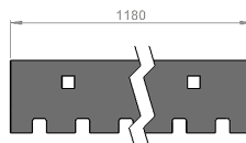
Tagget blad, slitesterkt stål 74131535 (tilleggsutstyr)
