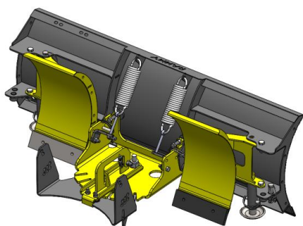
Bildet viser en plog med standardutstyr i transportstilling, bredde 118 cm
