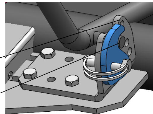
Frontmontert (1-rørs justerbar tilbehørsramme)
