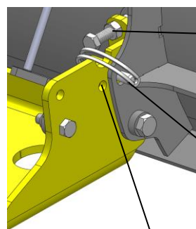
Mekanisk låsing av plogstøtdemper ved drift av kasteplag
