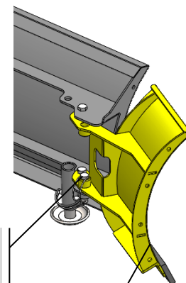
Vingene har 2 arbeidsstillinger og 1 transportstilling
