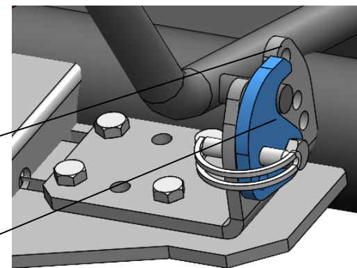
Etukiinnitys (1-putkinen)
