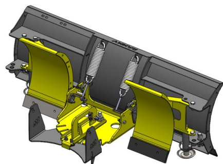
Kuvassa aura vakiovarusteilla kuljetusasennossa 118 cm leveänä
