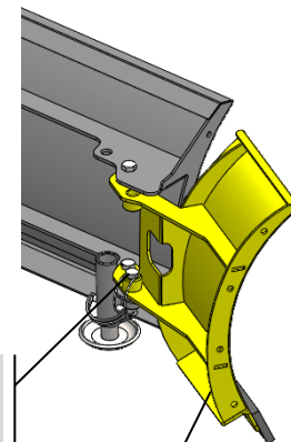
Siivissä 2 työasentoa ja kuljetusasento
