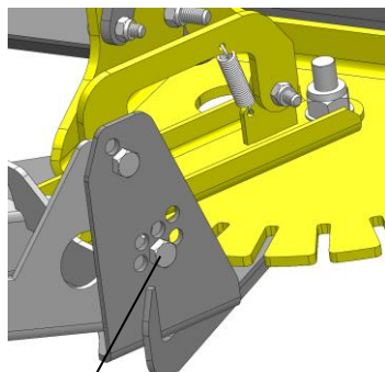
6-asentoinen kulman säätö
