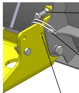
Auran iskunvaimennuksen mekaaninen lukitus Auralumilinkoa käytettäessä
